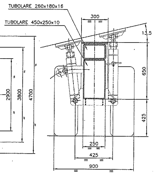
SEZIONE A-A SCALA 1:10
