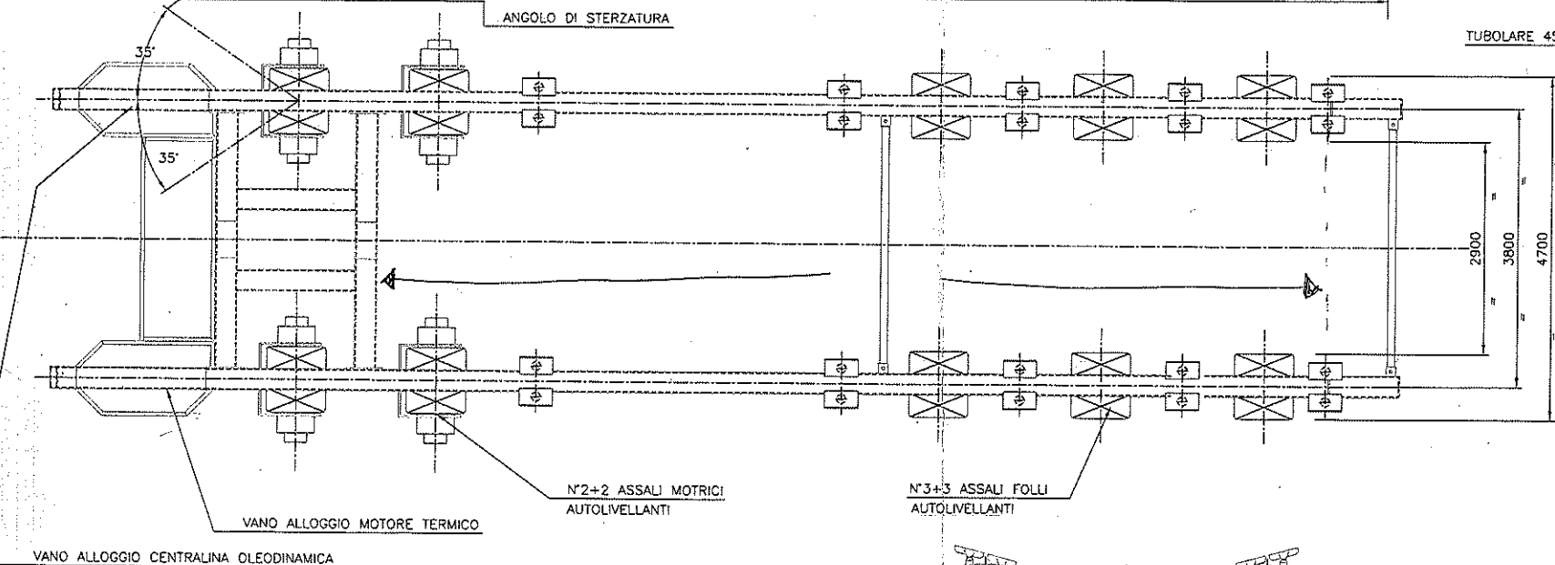
SEZIONE A-A SCALA 1:10
